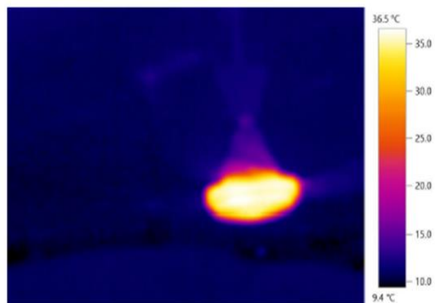
Thermal image of ceiling fan
